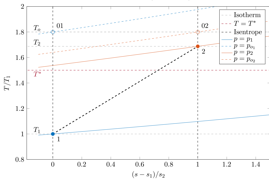
Normal shock ( Ts -diagram)
